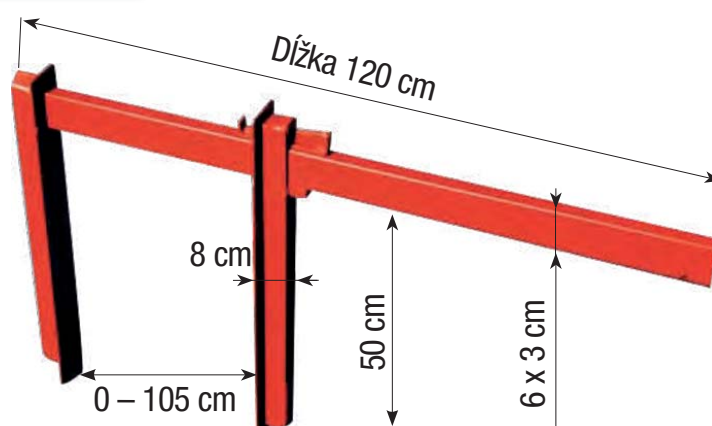
šalovacia zvierka základov
